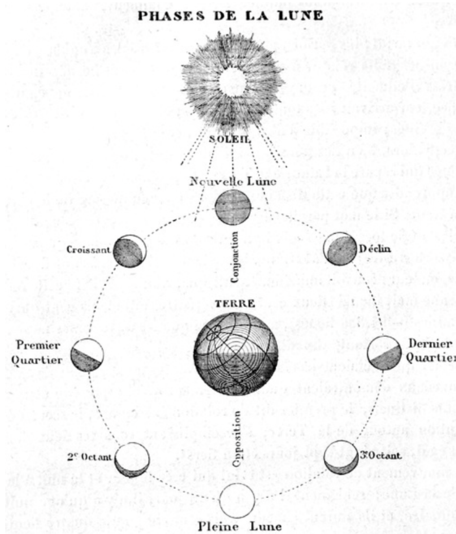
Figure 6 - Les mouvements de translation de la Lune
